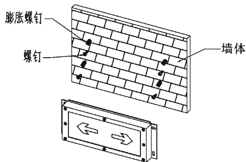
图 73 壁挂式单面标志灯具安装示意图
