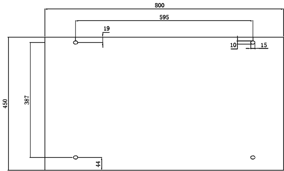
800*450*1400柜体底部安装孔位图
