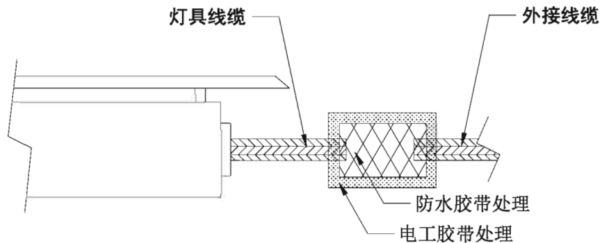
图 57 线缆接头密封示例
