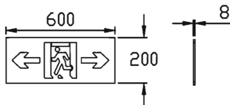
壁挂式大型单面标志灯具外形示意图
