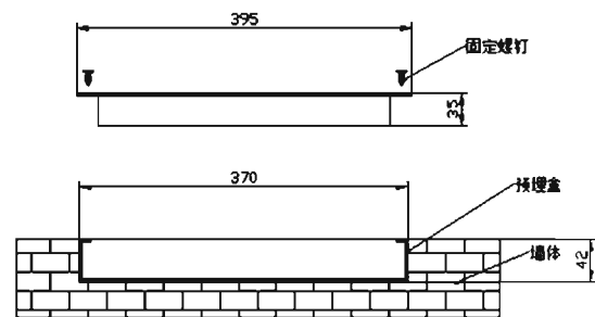
图 74 嵌入式单面标志灯具安装示意图
