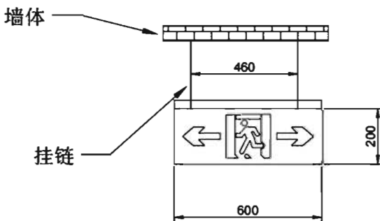
吊装式大型单面标志灯具安装示意图
