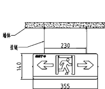
吊装式中型单面标志灯具安装示意图
