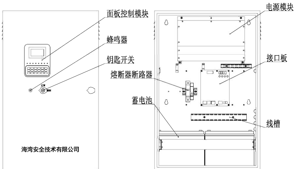
图 35 HW-D-0.3KVA-NF42/HW-D-0.5KVA-NF41
