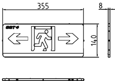
吊装式中型单面标志灯具外形示意图
