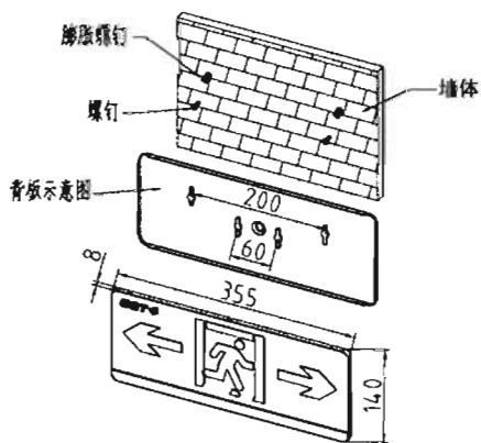
壁挂式中型单面标志灯具安装示意图
