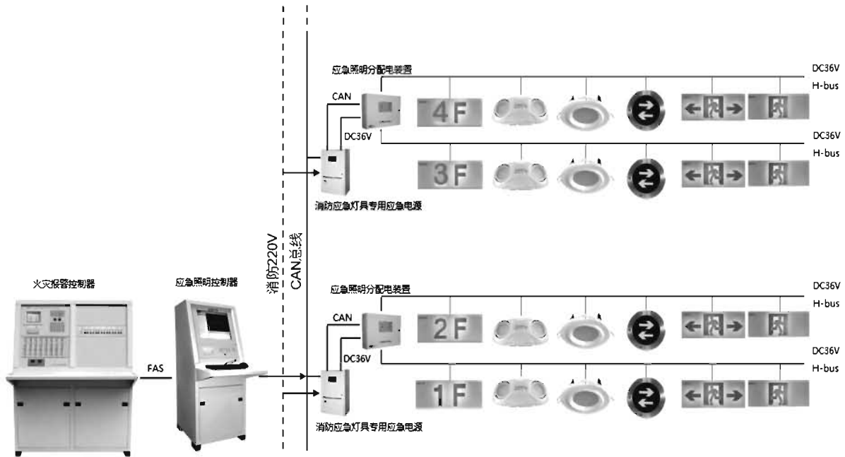
GST 海湾消防应急和疏散指示系统图 (分布式满足新设计规范)
