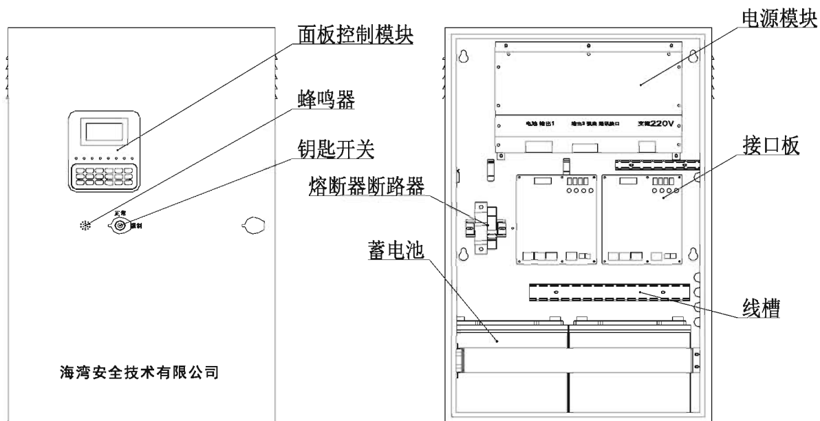
图 34 HW-D-0.5KVA-NF81
