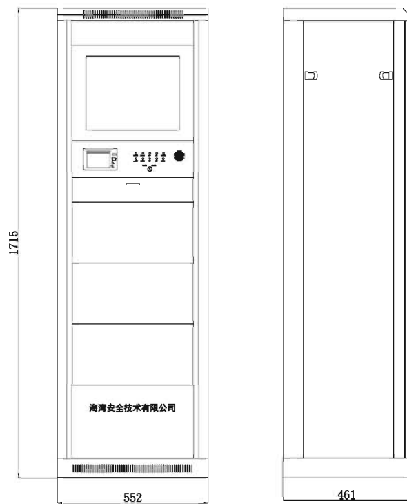
图 1 HW-C-60W-N100 结构
