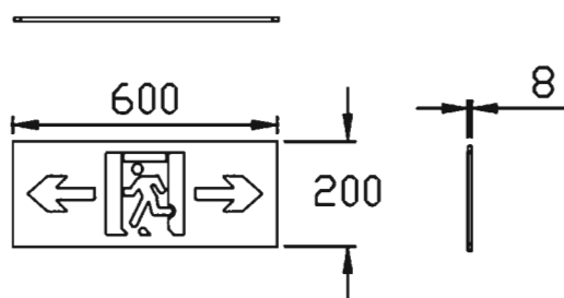
吊装式大型单面标志灯具外形示意图
