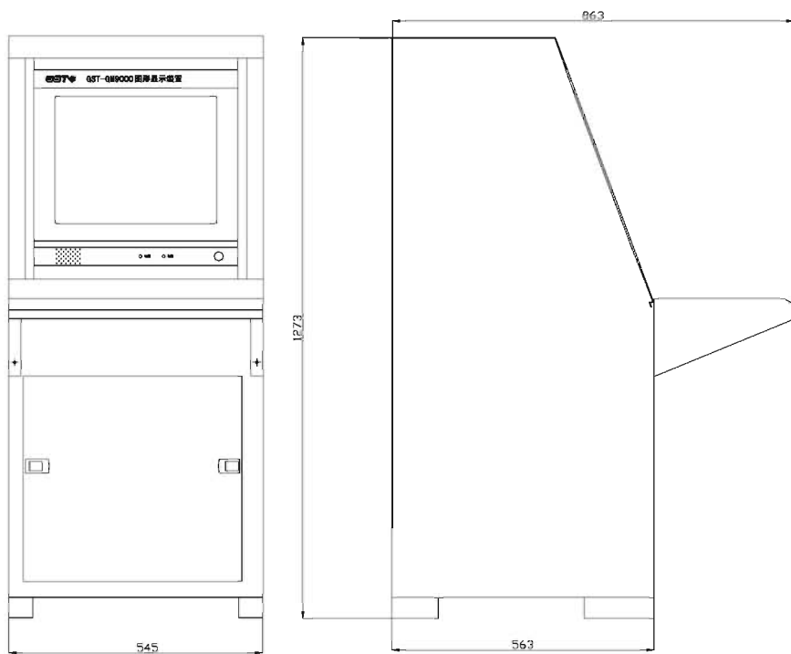
图 2 HW-C-60W-N110 结构
