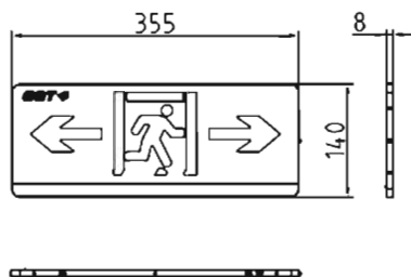
壁挂式中型单面标志灯具外形示意图
