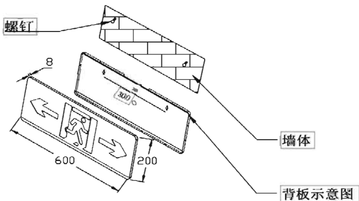
壁挂式大型单面标志灯具安装示意图
